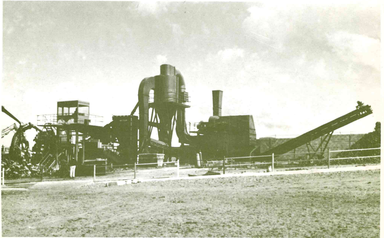
Planta de fragmentación Becker (sistema American Pulverizer) de automóviles y chapajo, de 1.000 CV. de potencia. Producción 16 t/h., instalada en la empresa de don Daniel González Riesta, de Gijón.
