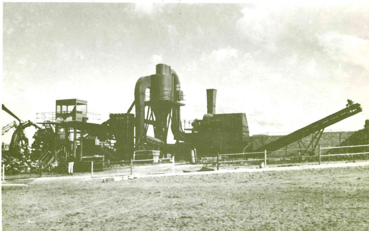
Planta de fragmentación Becker (sistema American Pulverizer) de automóviles y chapajo, de 1.000 CV. de potencia. Producción 16 t/h., instalada en la empresa de don Daniel González Riesta, de Gijón.
